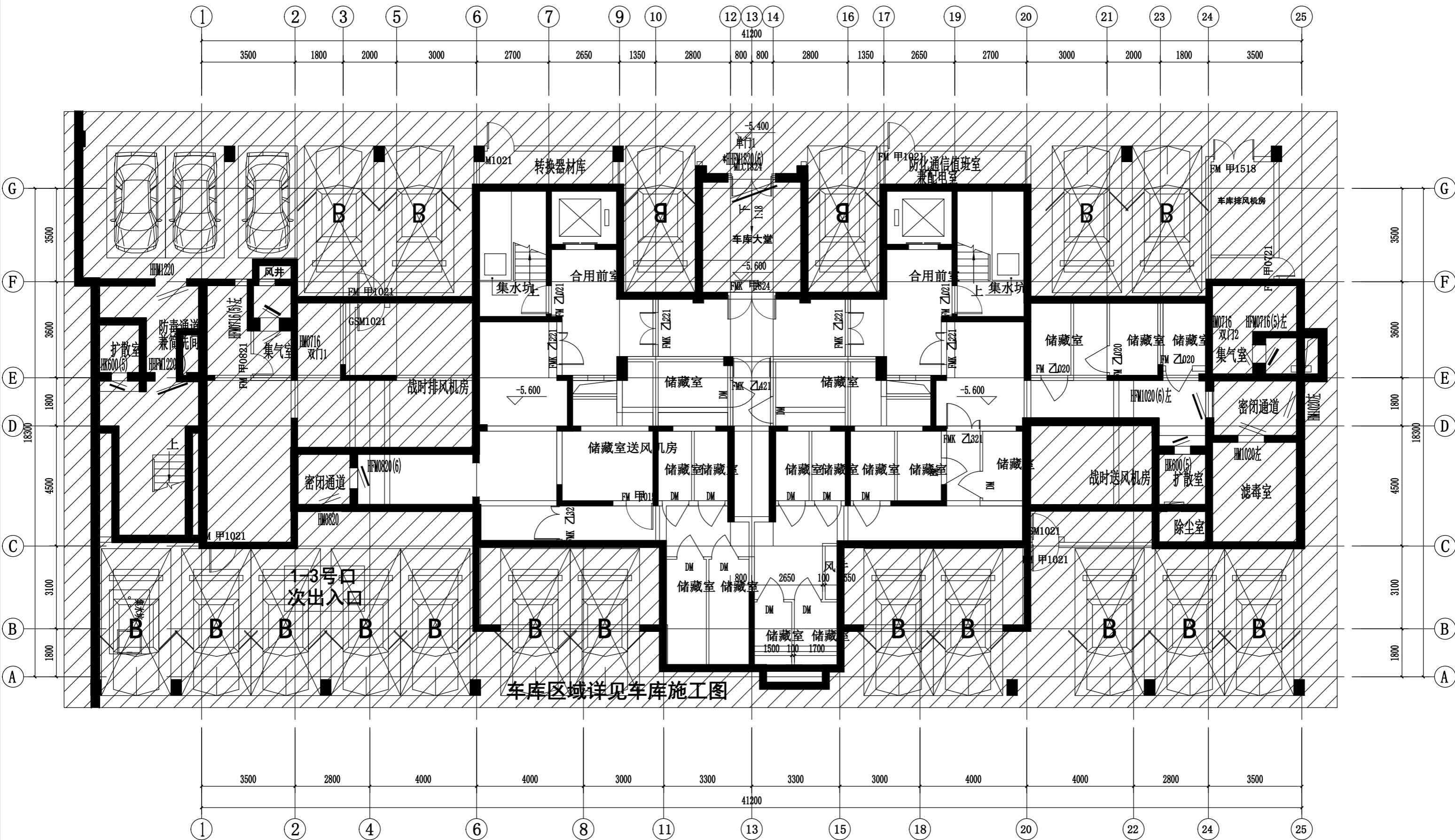
地下二层平面图
